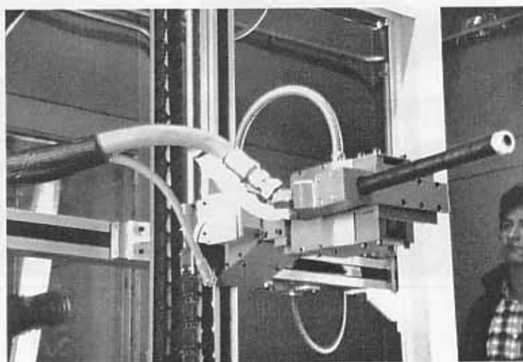
图2: 喷枪操纵器 (本图由华东泰克西汽车 铸造有限公司提供)
